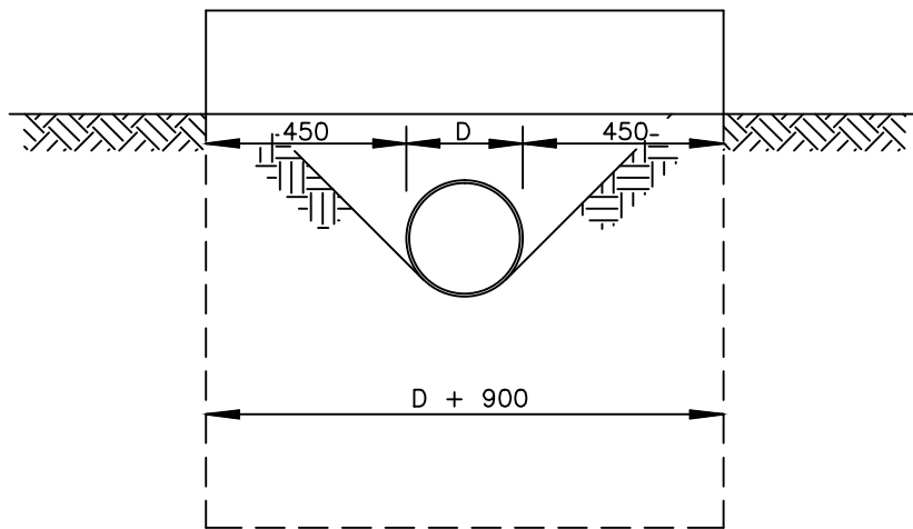
END ELEVATION
