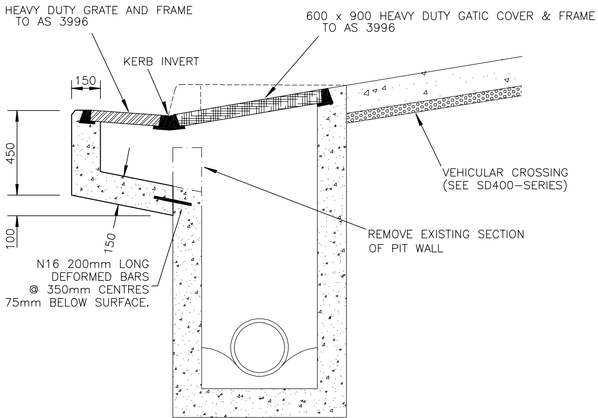
SECTION A-A
